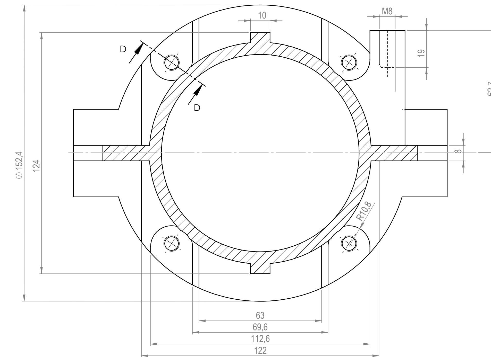
KESİT E-E ÖLÇEK 1 : 1
