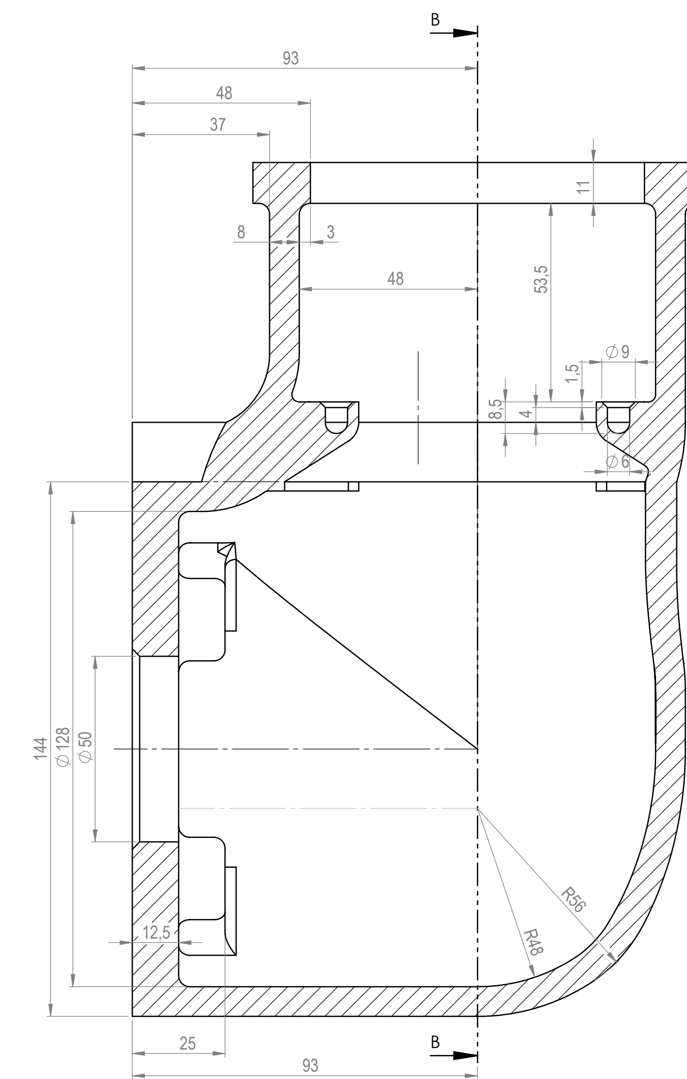
KESİT A-A
