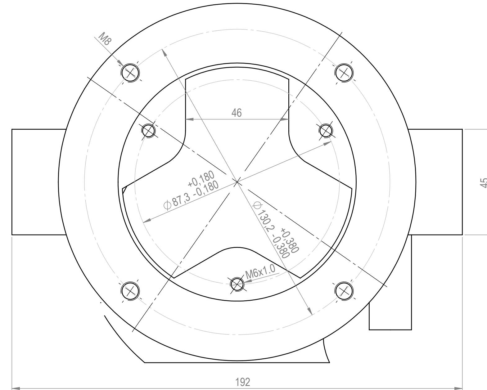
GÖRÜNÜM C ÖLÇEK 1 : 1
