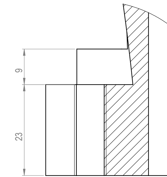
KEŞİT DETAIL D ÖLÇEK 2 : 1
